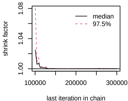
d.I.II
