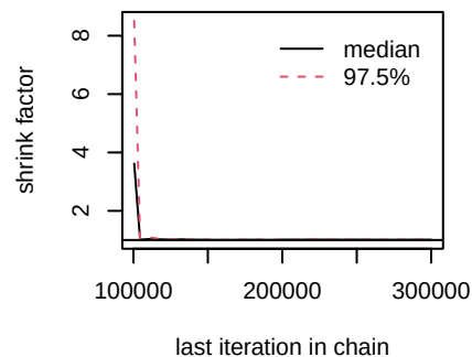
d.I.I_MMPi
