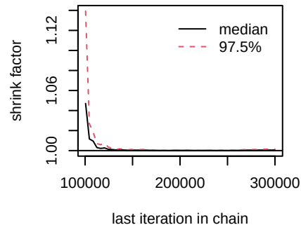
d.III.III_antiangio
