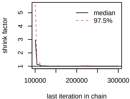
d.I.I_PARPi
