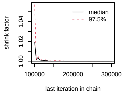
d.I.I_antiangio
