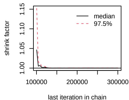
d.I.III
